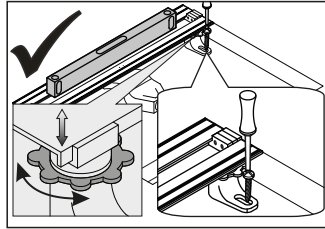
Kanalı zemine yerleştirin.
