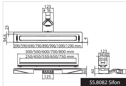
SS.8082 Sifon
