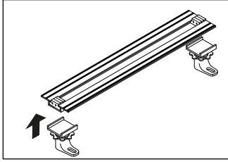
Yükseklik ayar parçasını gövdeye yerleştirin.
